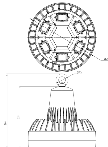
Рисунок 2. Габаритный чертеж
