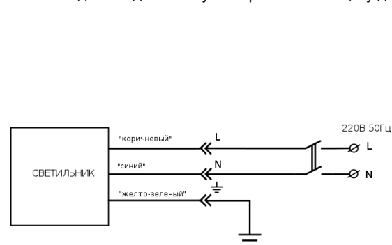
Рисунок 1. Электрическая схема подключения.
