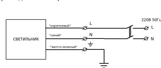
Рисунок 1. Электрическая схема подключения.
