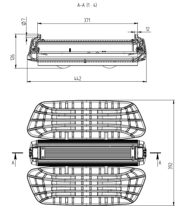
Рисунок 2. Габаритный чертеж
