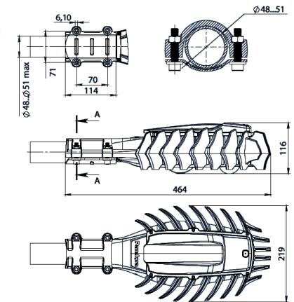
Рисунок 3. Габаритный чертеж
