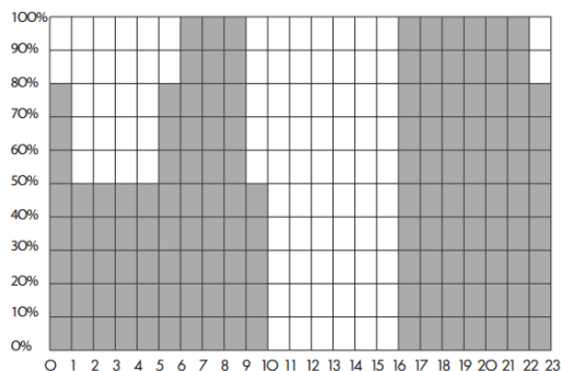
Рисунок 4. Предустановленный заводской суточный график
