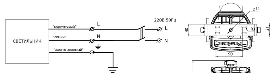
Рисунок 1. Электрическая схема подключения.
