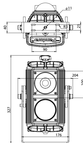
Рисунок 2. Габаритный чертеж
