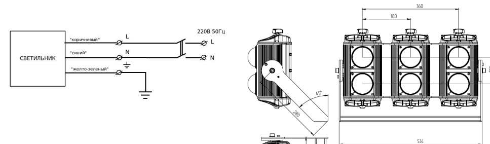
Рисунок 1. Электрическая схема подключения.
