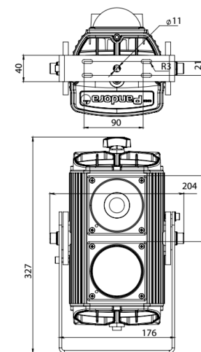
Рисунок 2. Габаритный чертеж
