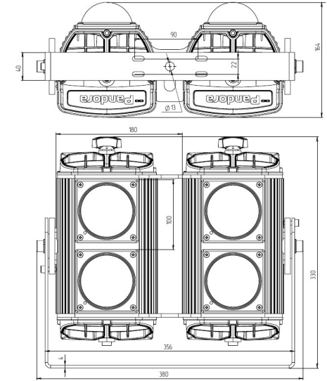
Рисунок 2. Габаритный чертёж
