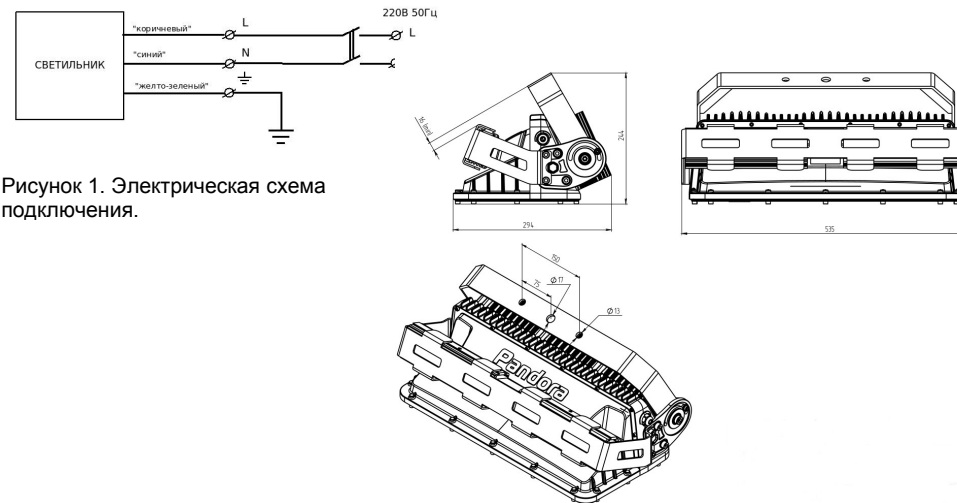
Рисунок 2. Габаритный чертеж
