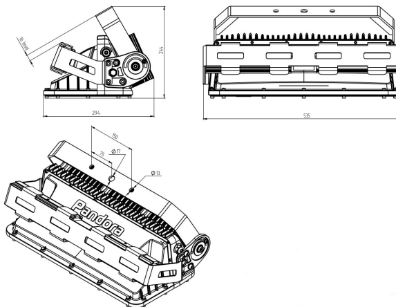
Рисунок 2. Габаритный чертёж
