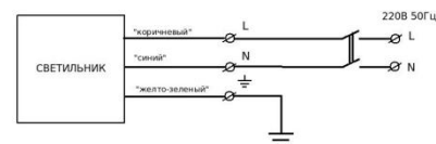
Рисунок 2. Электрическая схема подключения
