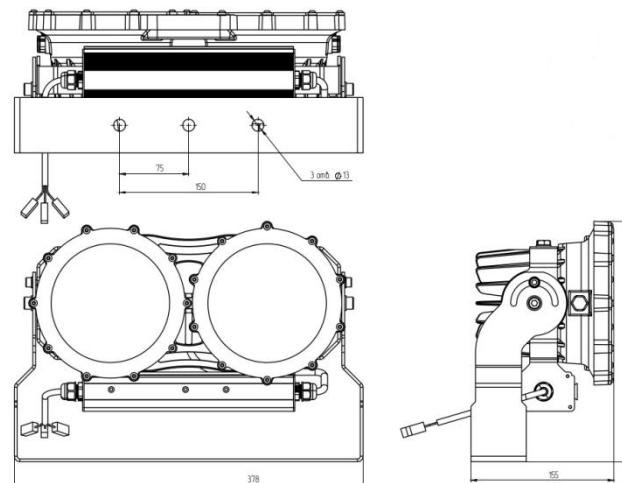
Рисунок 1. Габаритный чертеж
