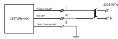
Рисунок 2. Электрическая схема подключения
