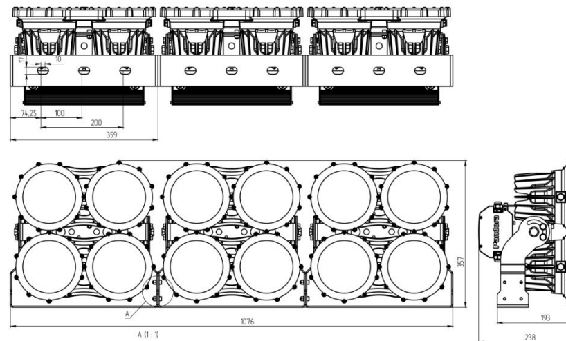
Рисунок 1. Габаритный чертеж
