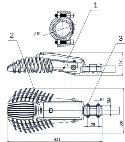
Рисунок 2. Схема установки светильника на кронштейн.
