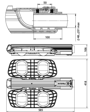
Рисунок 3. Габаритный чертёж
