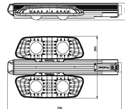
Рисунок 3. Габаритный чертеж
