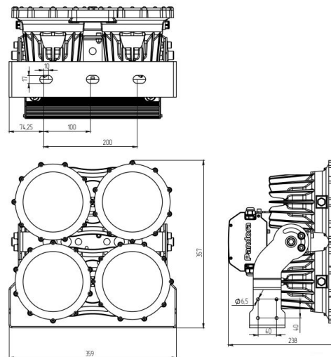
Рисунок 1. Габаритный чертеж
