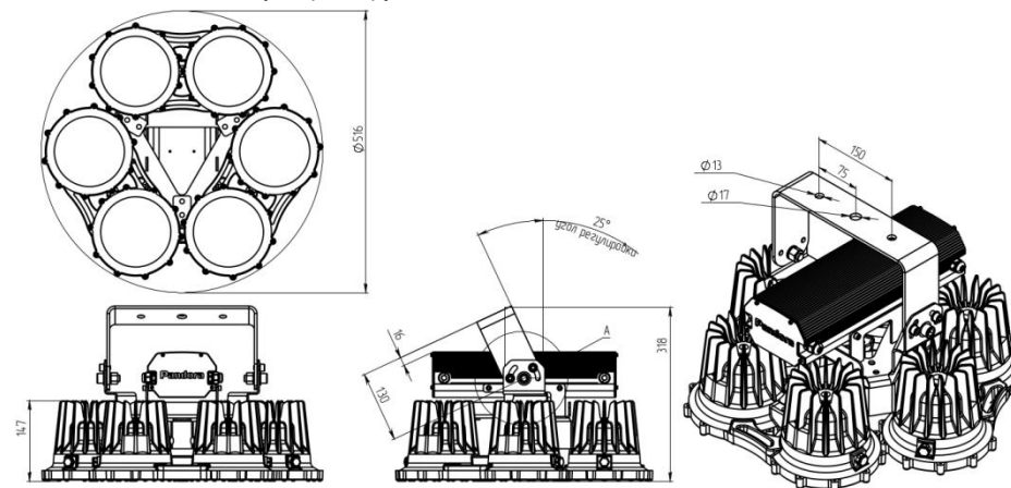
Рисунок 1. Габаритный чертеж
