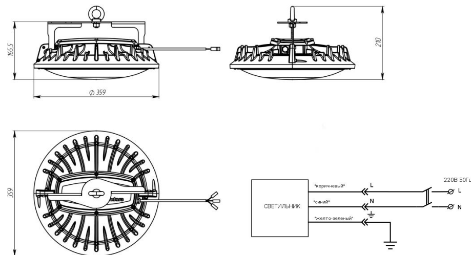
Рисунок 1. Габаритный чертеж.
