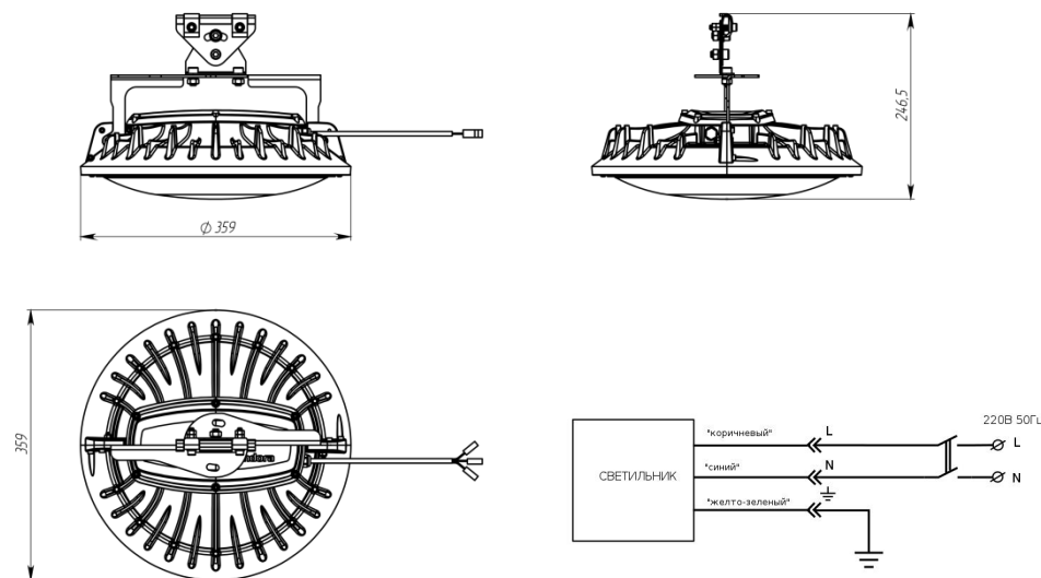
Рисунок 1. Габаритный чертеж.
