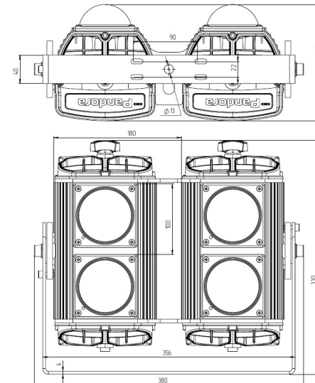
Рисунок 2. Габаритный чертеж
