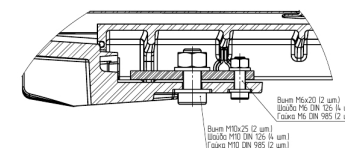
Рисунок 2. Габаритный чертеж
