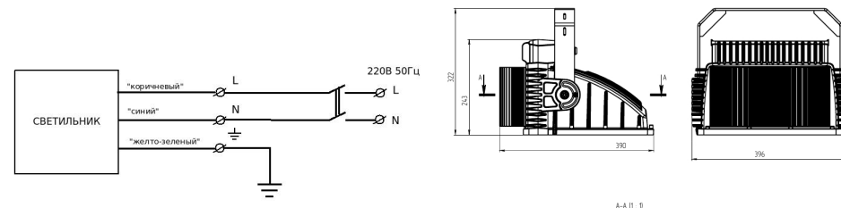
Рисунок 1. Электрическая схема подключения.
