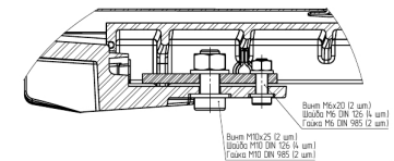
Рисунок 2. Габаритный чертеж
